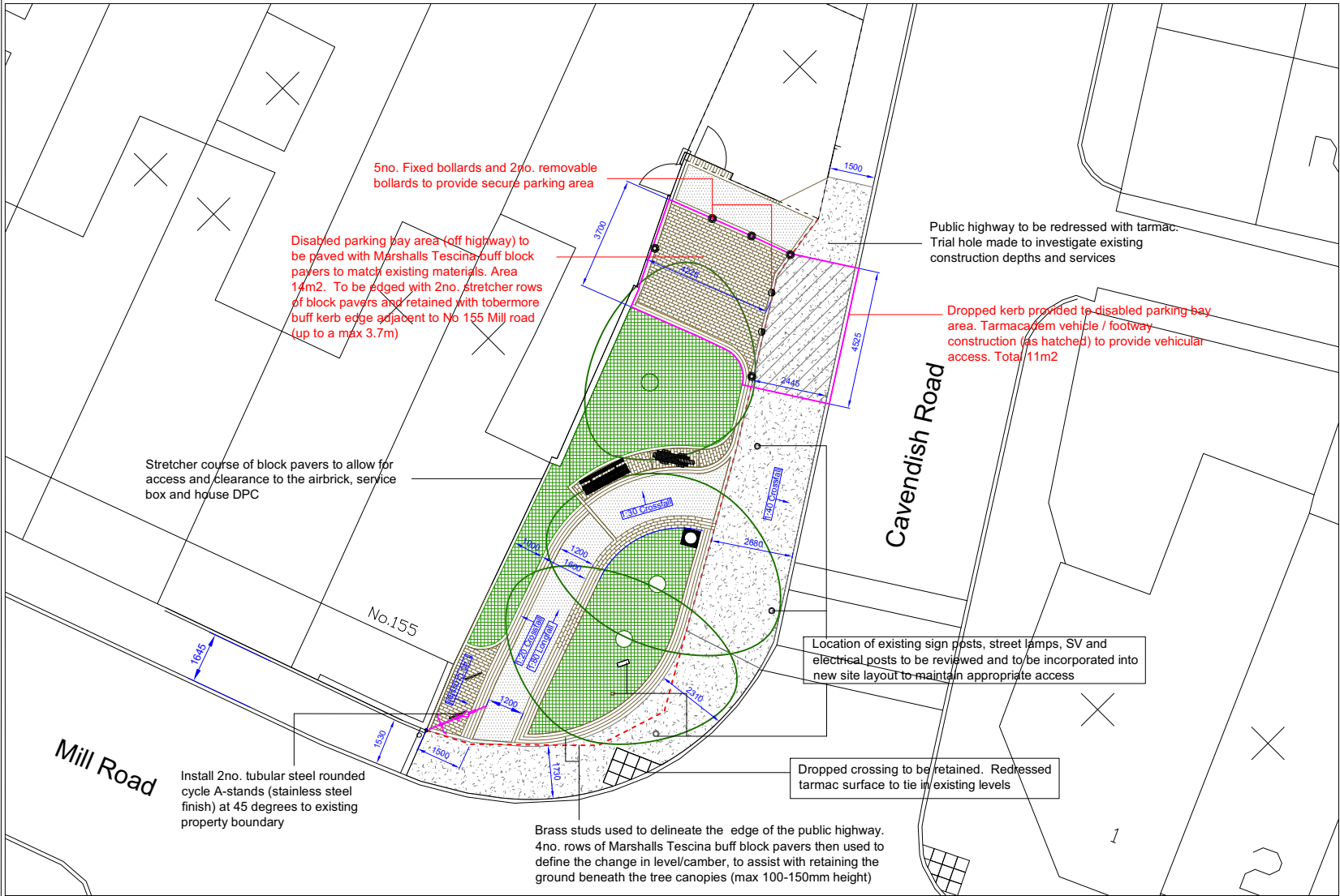
Plan 1:100 @A2
